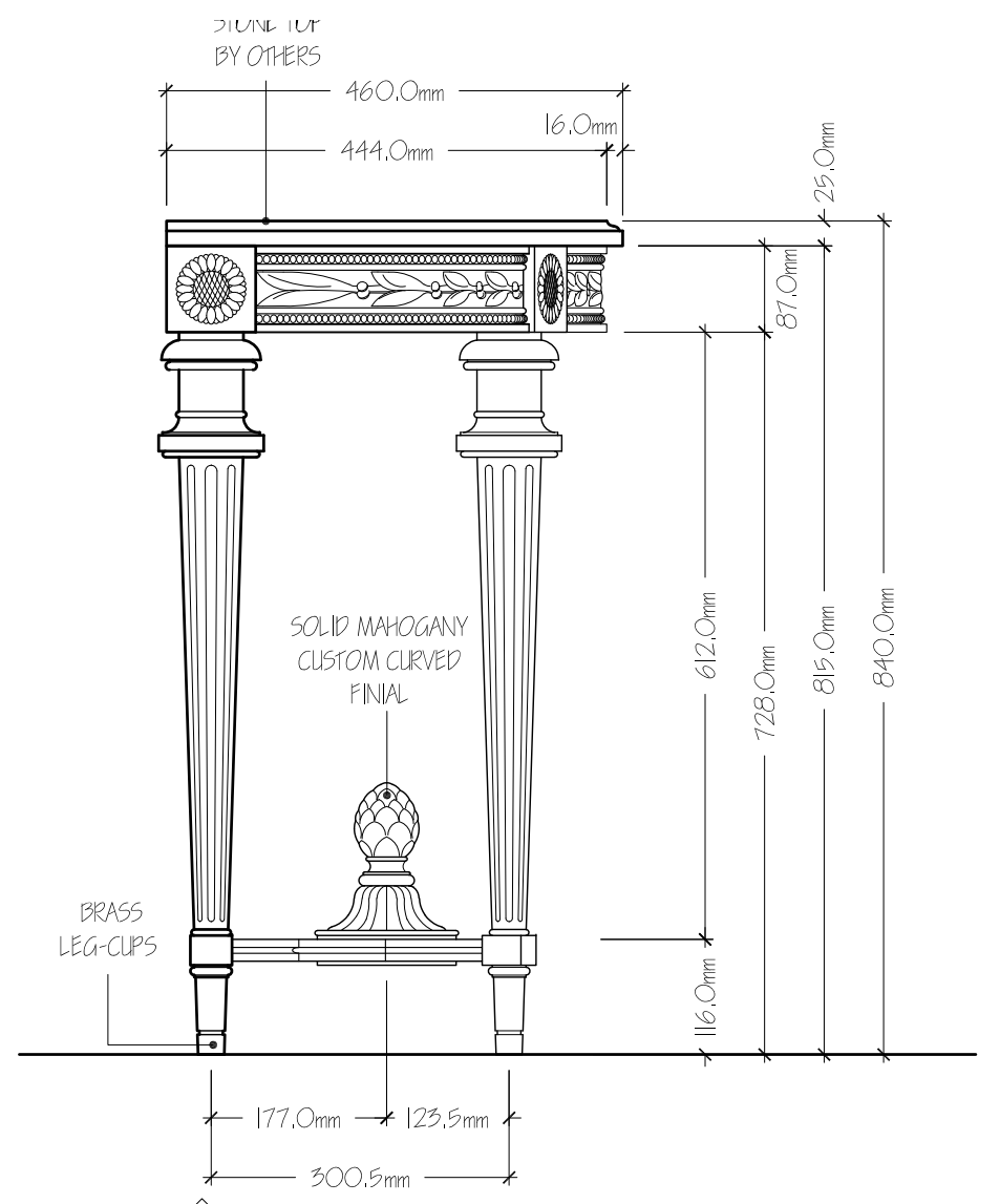
ELEVATION SCALE: 1:8
