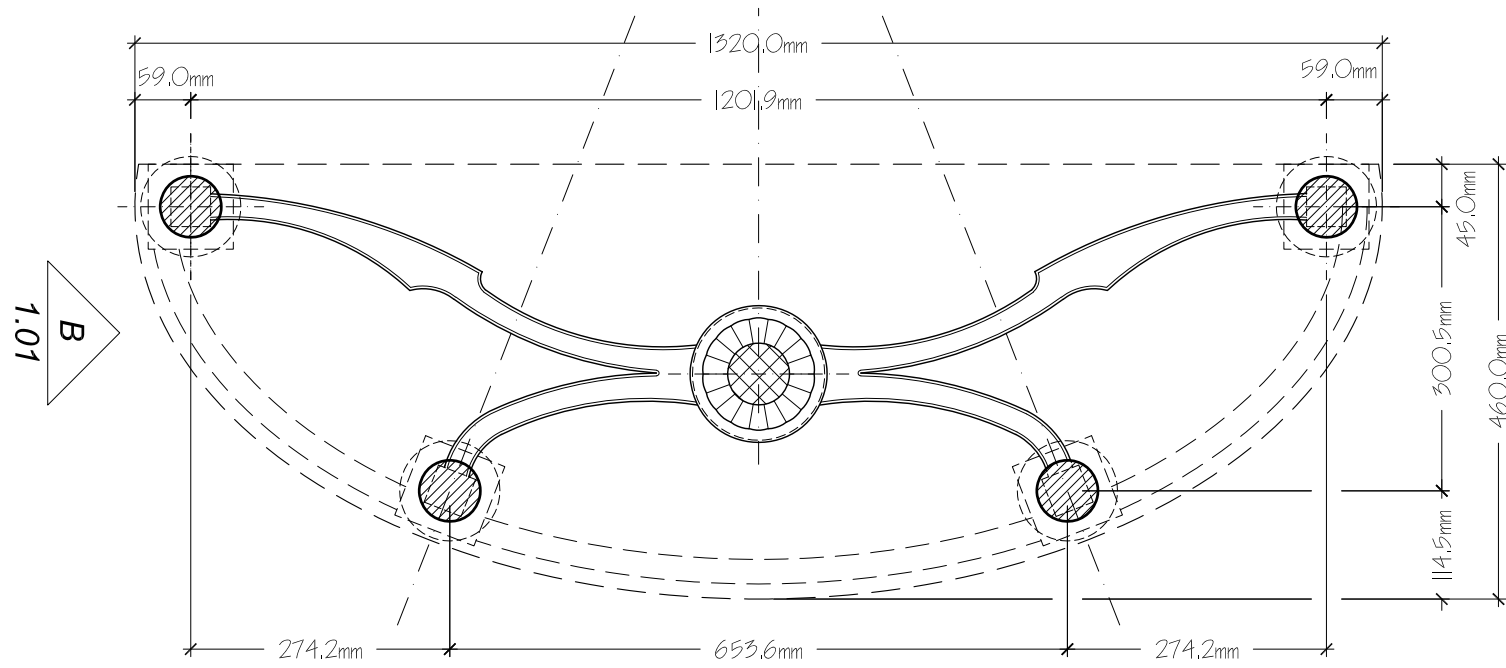
PLAN SCALE: 1:8
