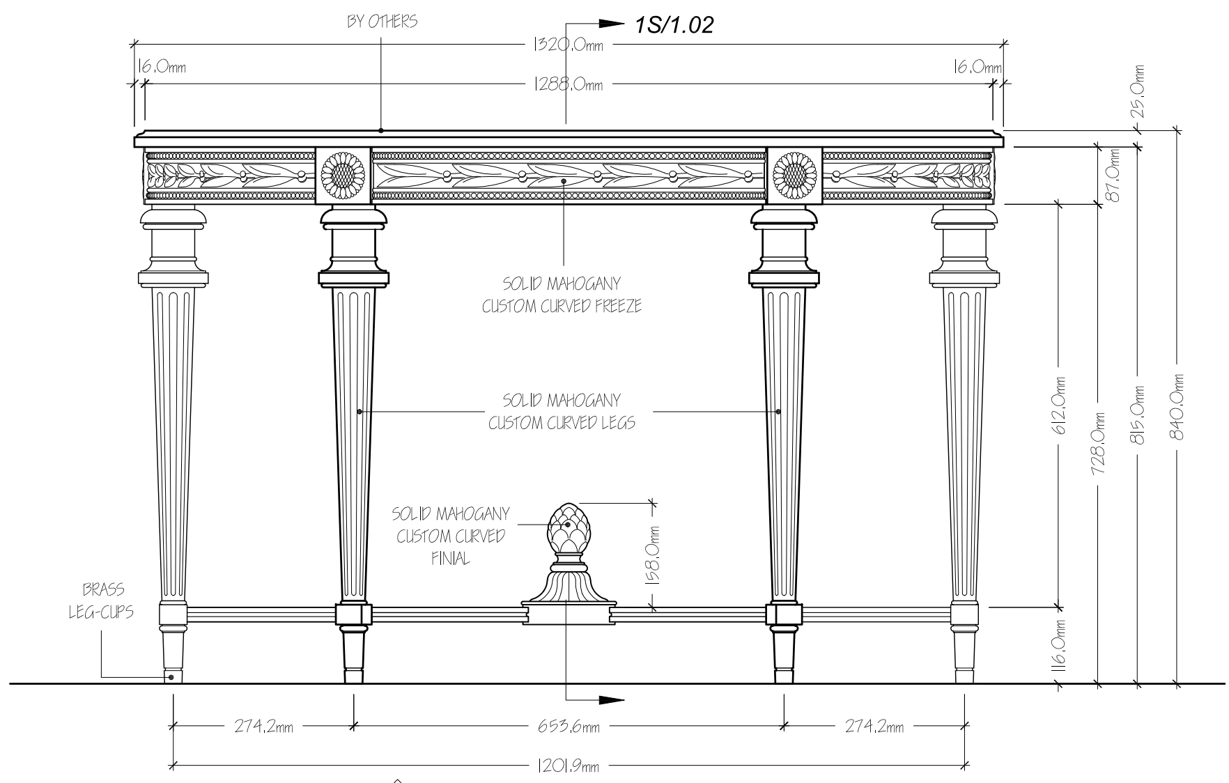
ELEVATION SCALE: 1:8
